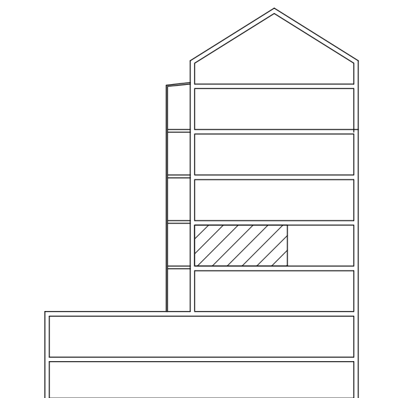
PRINCIPSEKTION
